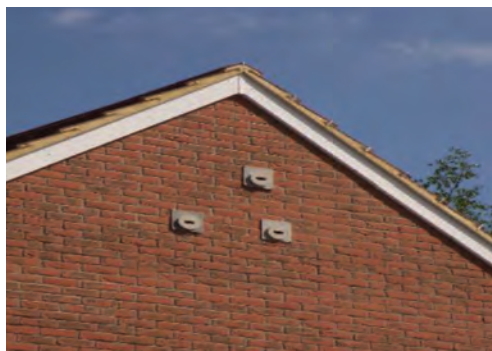
Fot. 114. Niemal niewidoczna skrzynka wewnętrzna chroniona przed warunkami atmosferycznymi może być wykonana z cienkiej i taniej sklejk. Do jej wnętrza prowadzi chropowata, ułatwiająca zwierzętom dostawanie się do wewnątrz rura PCV poprowadzona przez warstwę termoizolacyjną oraz ścianę (DN)
