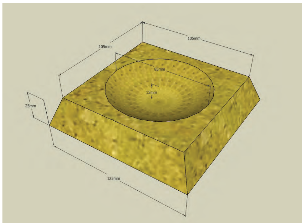
Fot. 123. Wymiary niecki gniazdowej dla jerzyków (DN)
